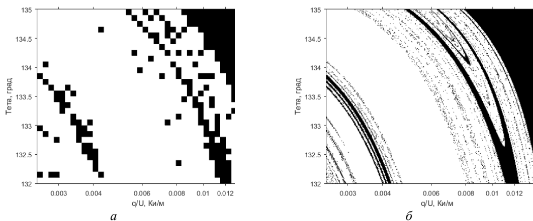
Рис. 4. Области выбора начальных значений q/U и 2 , при которых численный алгоритм сходится к оптимальным значениям для периода А: а – «грубая» сетка; б – «мелкая» сетка.
